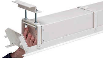
Revisionsklappe offen
