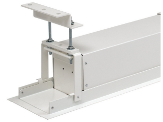
Revisionsklappe geschlossen
