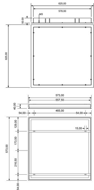
Einbaurahmen
