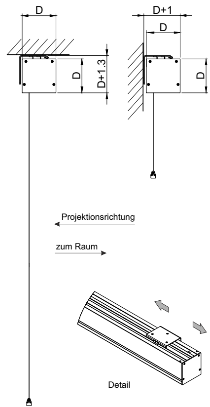
Deckenmontage
